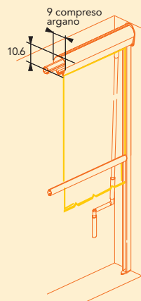
TF 0G Il cassonetto, compreso l'occhiolo dell'argano ha ingombro massimo di cm 9 in profondità e cm 10,6 in altezza
