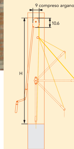
TF 4 Il cassonetto, compreso l'occhiolo dell'argano ha ingombro massimo di cm 9 in profondità e cm 10,6 in altezza
